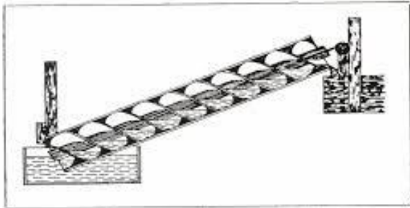
38. Το αρχαίο ξύλινο Αρχιμήδη, μηχανισμός για την άντληση νερού. Γραμμική ανατομία από τον L. Sprague de Camp.
